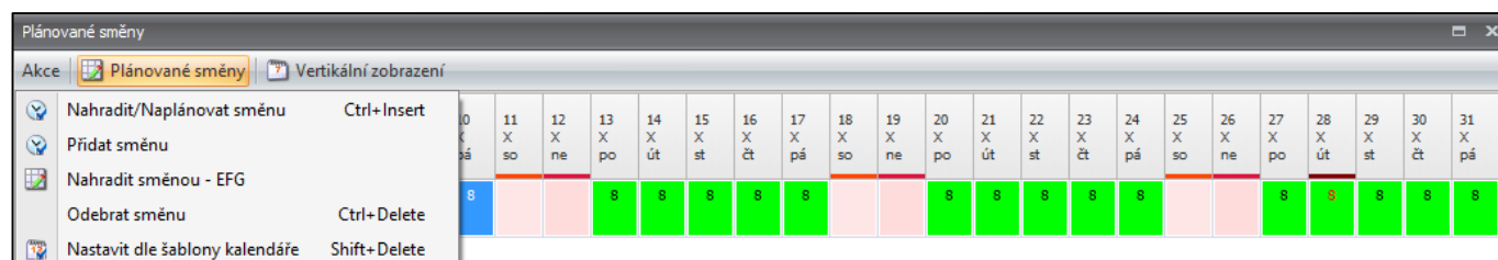
Obr. 3: Nabídka Akce
